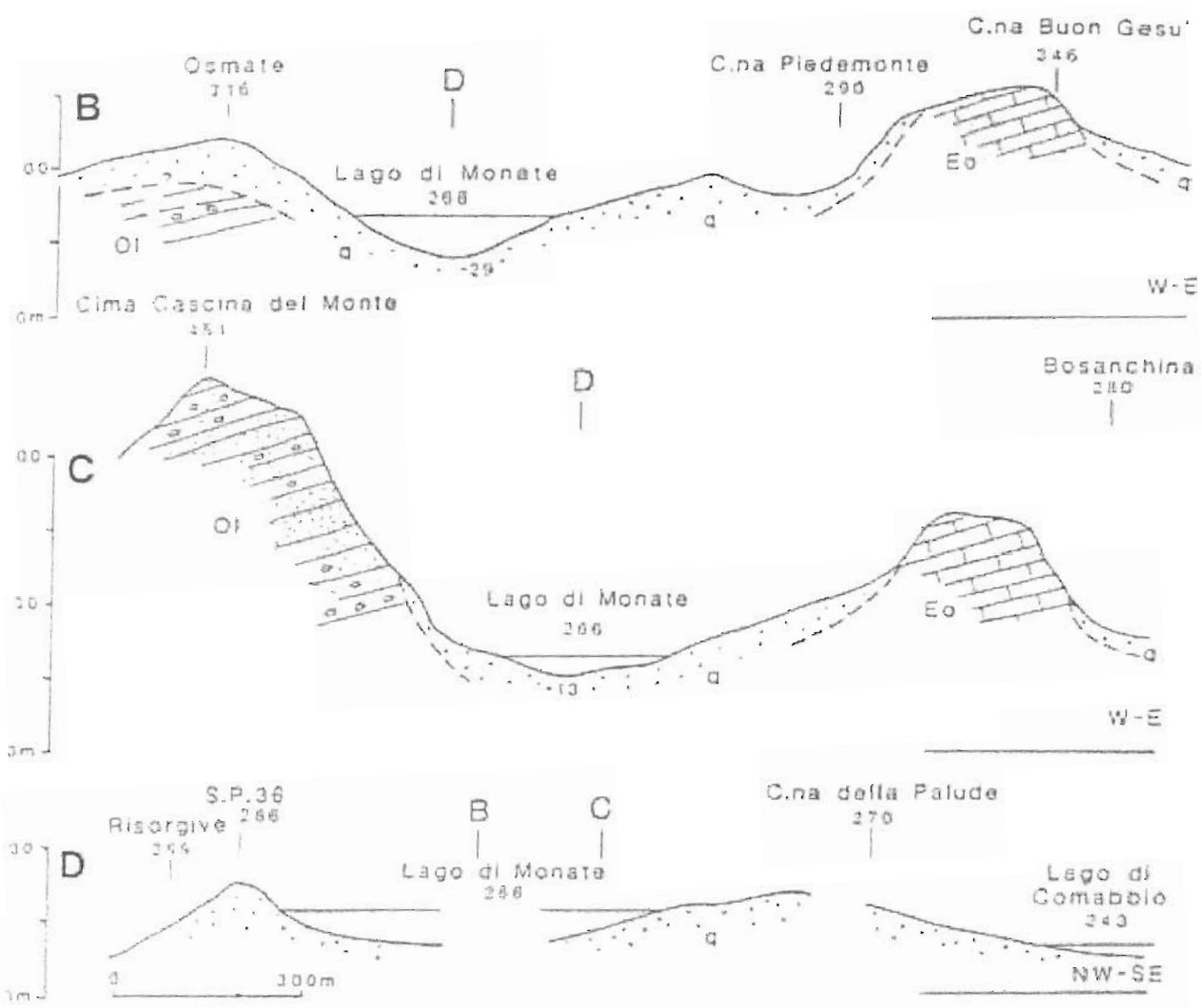
Sezioni geologiche B, C, D. (tracce delle sezioni in fig. 3). q = Quaternario (lacustre e morenico); Ol = Oligocene ( gonfolite ); Eo = Eocene ( Calcarei Nummulitici ).
