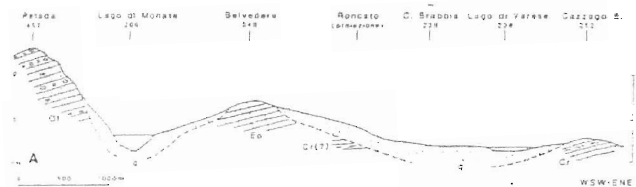
1. Sezione geologica A: M. Pelada-Cazzago Brabbia (traccia della sezione in fig. 1). q = Quaternario (lacustre e (terico), Ol = Oligocene ( Gonfolite ); Eo = Eocene ( Calcarei Nummulitici ); Cr = Cretaceo ( Flysch ).
